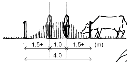
doorsnede maatvoering
